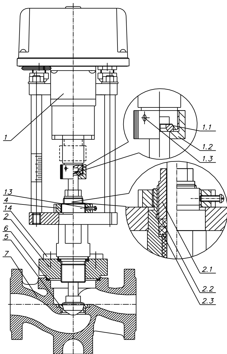
Рисунок 1 Общее устройство клапана КЗР 25/XX.В
