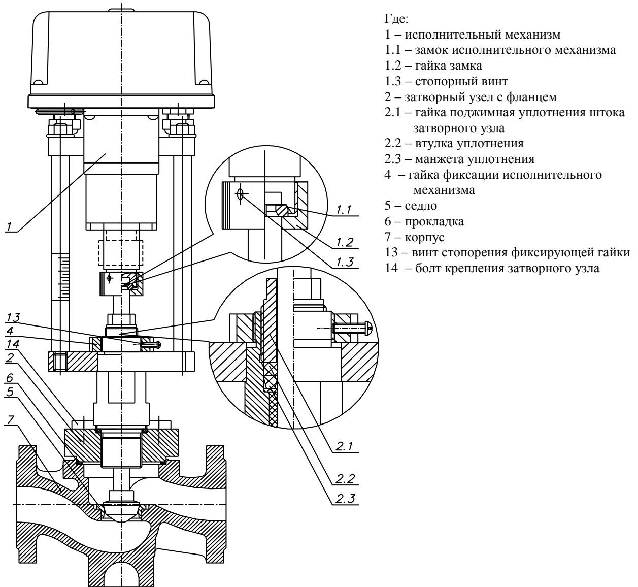
Рисунок 1. Общее устройство клапана КЗР 50/XX.B
