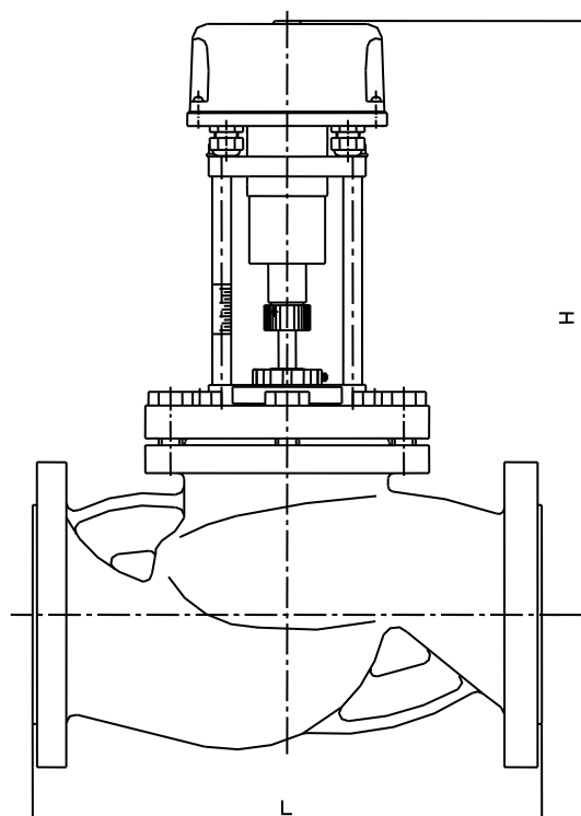
Рисунок 1. Общий вид клапана
