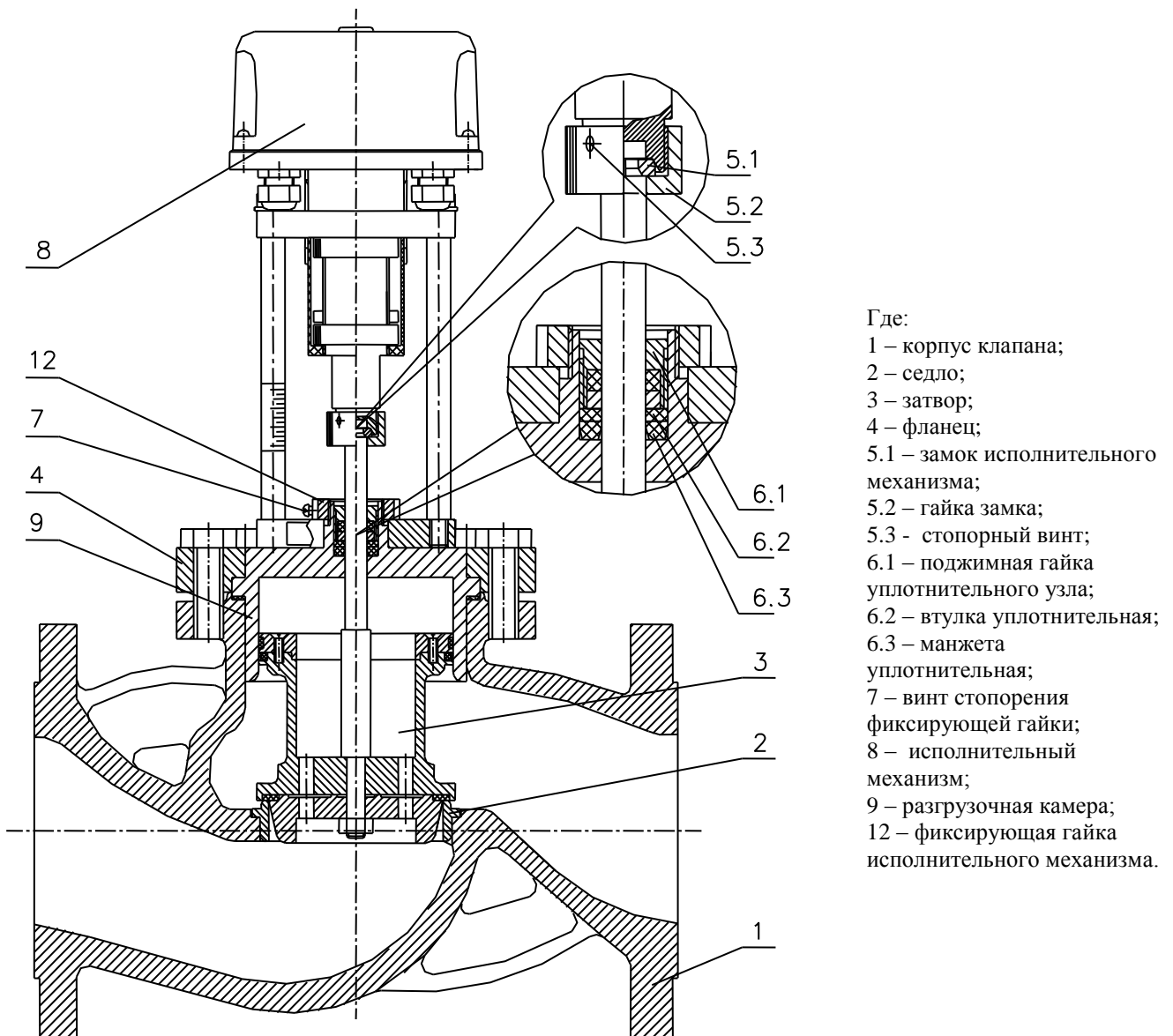
Рисунок 1 Общее устройство клапана КЗРр-100/95.В
