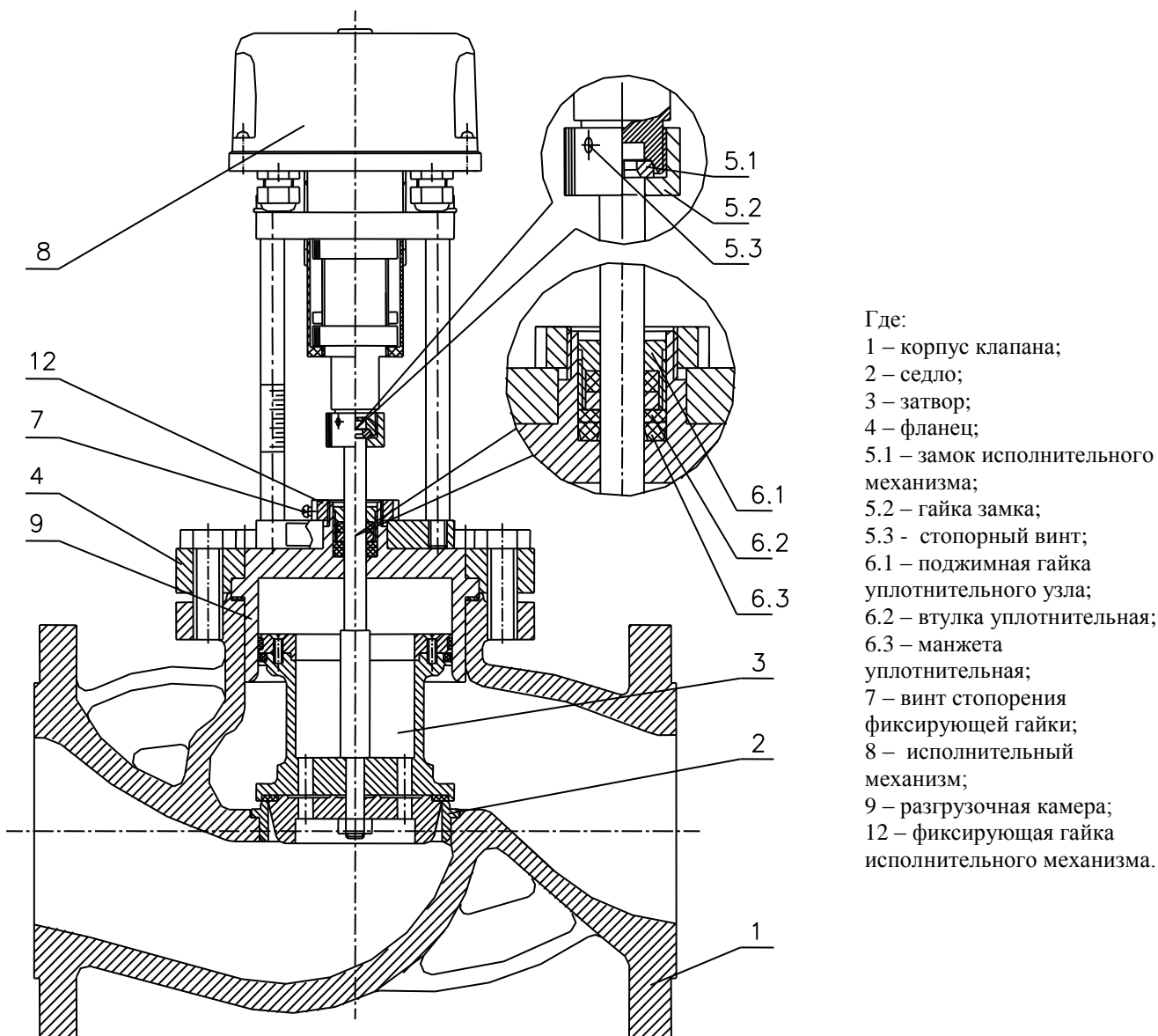
Рисунок 1. Общее устройство клапана КЗРр-125/120.Б-XX
