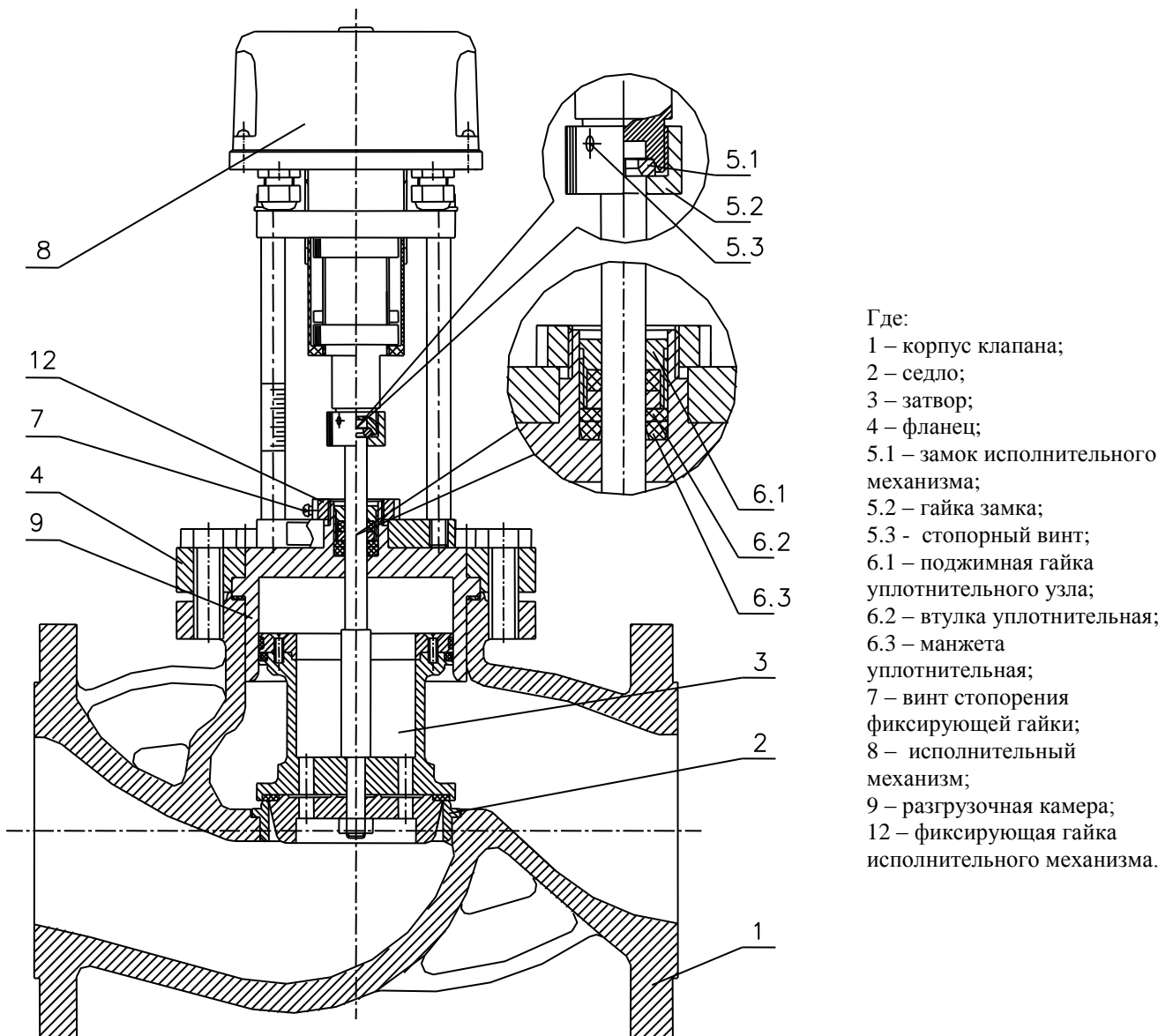
Рисунок 1. Общее устройство клапана КЗРр-125/120.В
