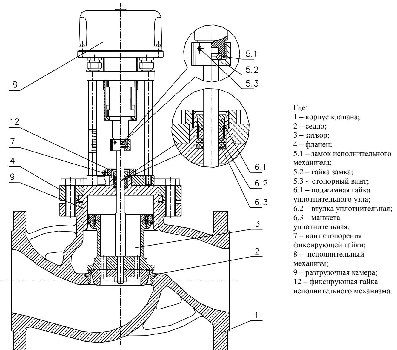
Рисунок 1. Общее устройство клапана КЗРр-150/145.Б-XX
