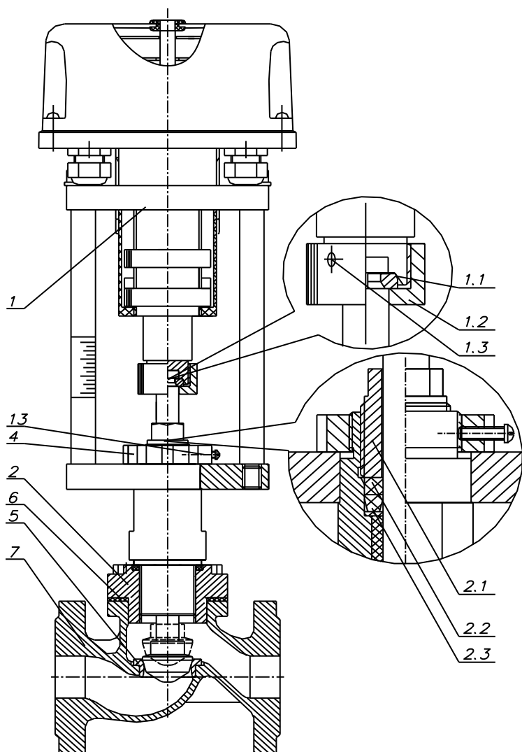
Рисунок 1. Общее устройство клапана КЗР-20/XX.B
