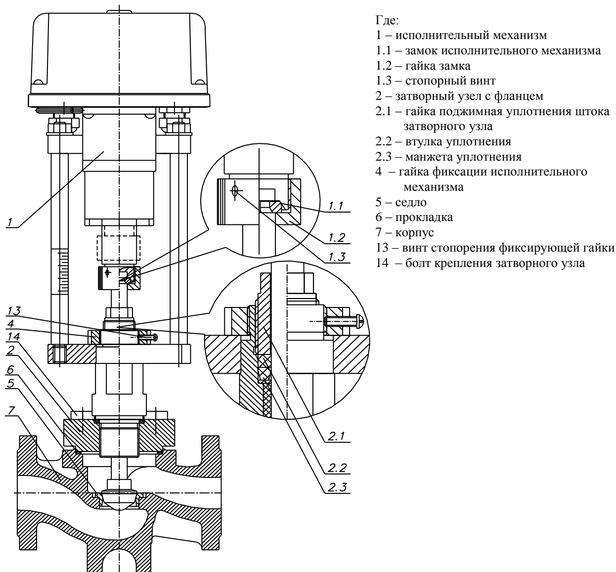
Рисунок 1 Общее устройство клапана КЗР 32/31,5.Б-ХХ
