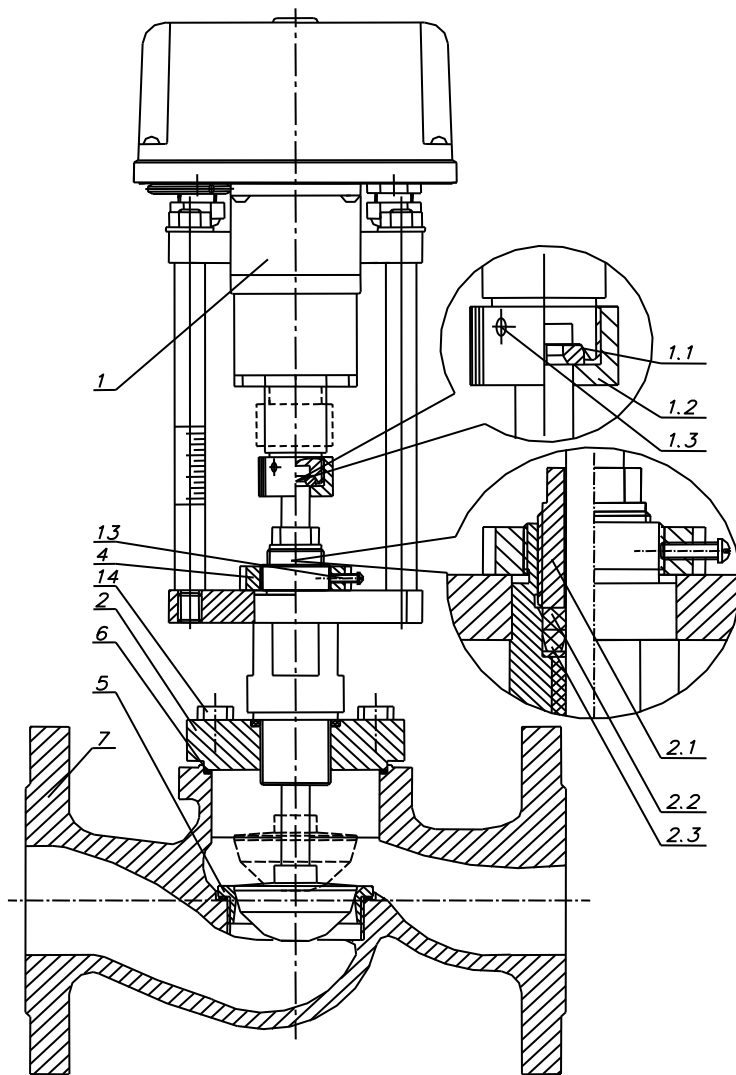
Рисунок 1. Общее устройство клапана КЗР - 40/40.В
