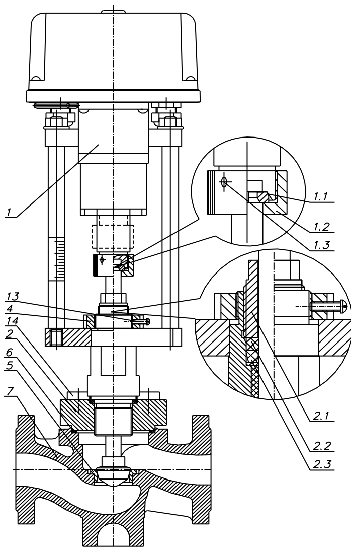
Рисунок 1. Общее устройство клапана КЗР - 80/76.Б-XX
