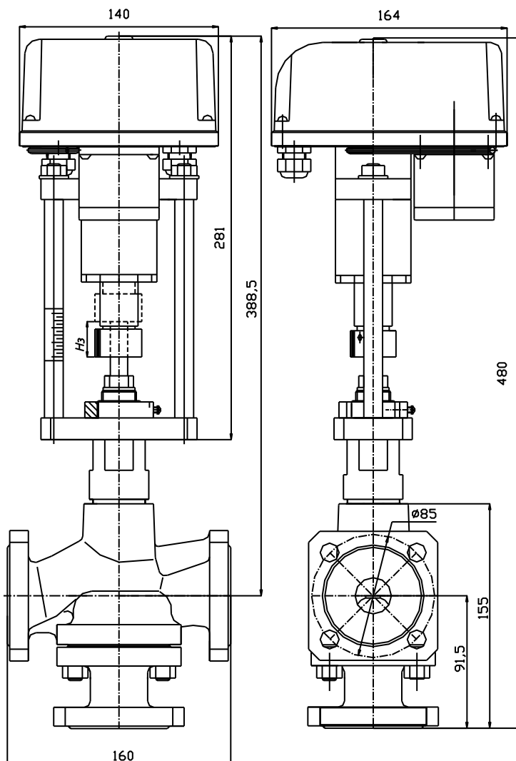
Рисунок 1. Общий вид клапана
