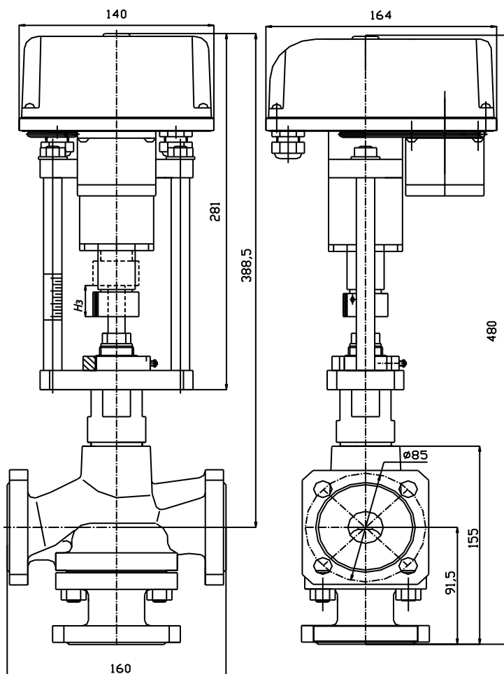
Рисунок 1. Общий вид клапана
