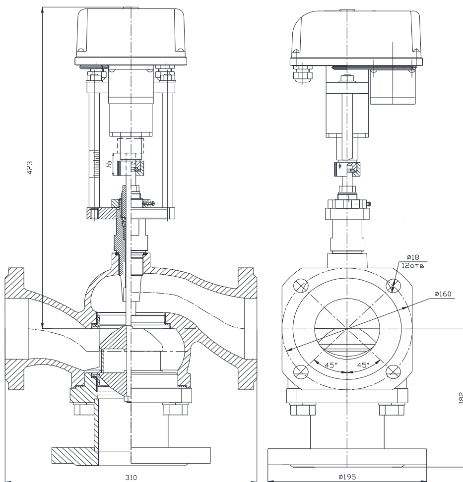
Рисунок 1. Общий вид клапана
