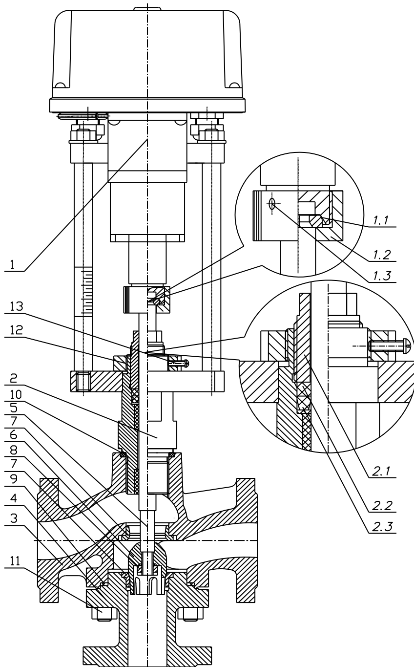
Рисунок 1 Общее устройство клапана смесительного трехходового КСТ-40/XX.B
